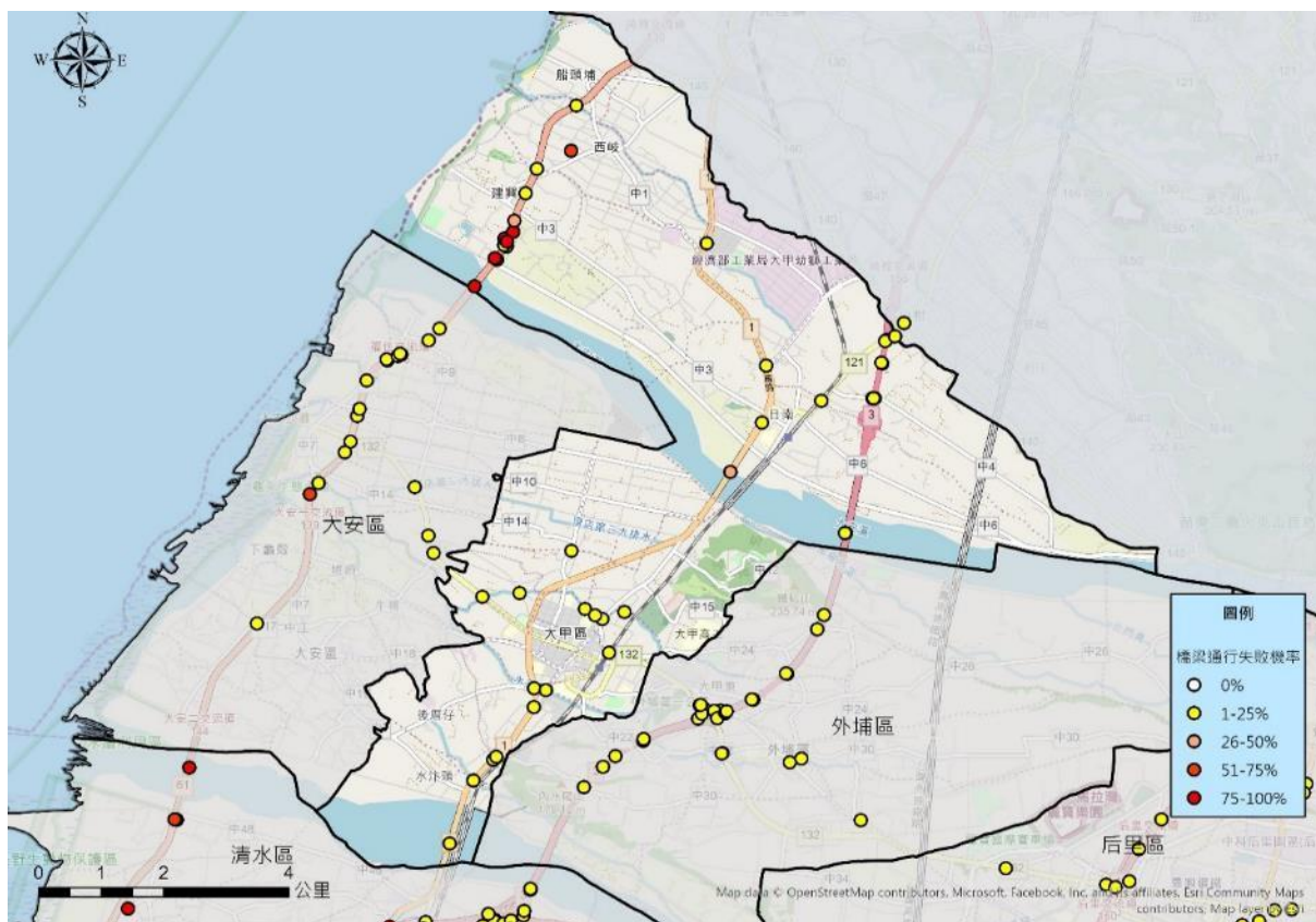
圖 1-3-8 大甲區受損橋梁分布圖
