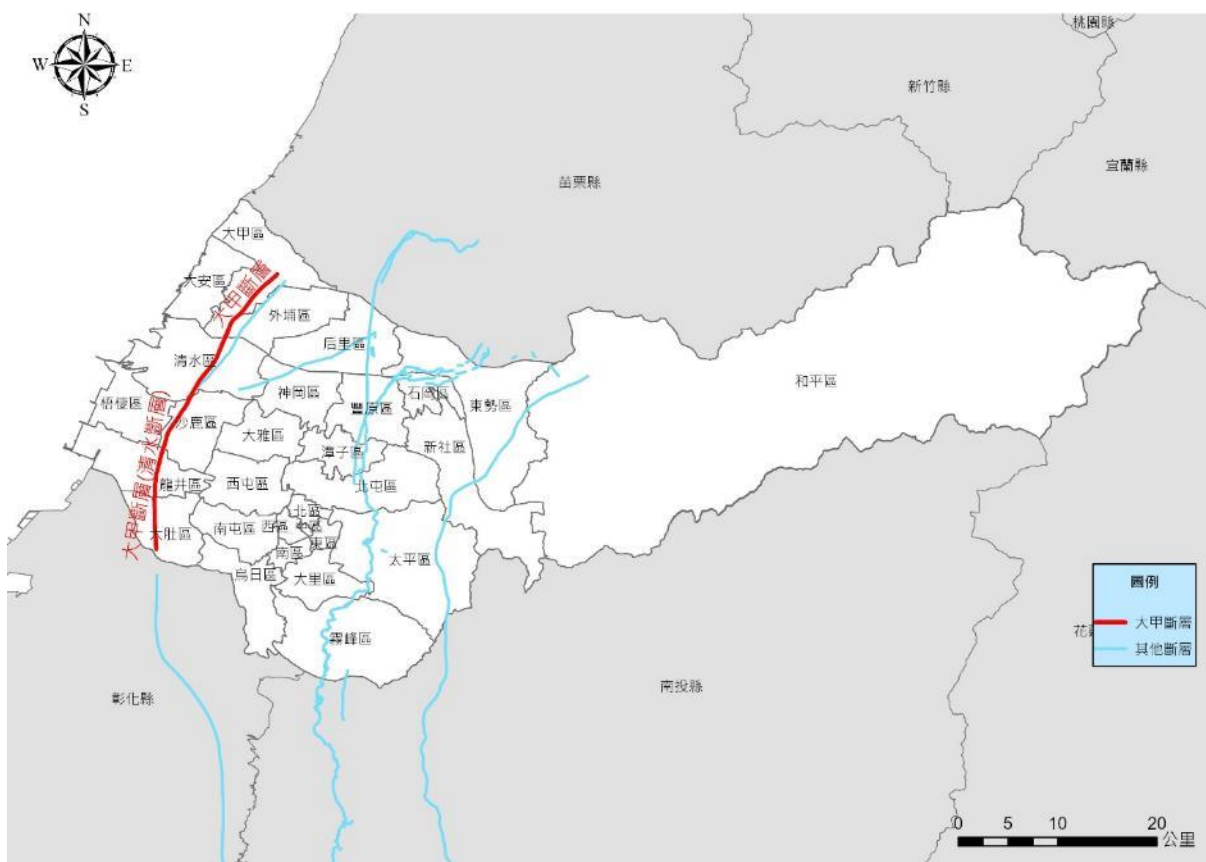
圖 1-3-4 大甲區斷層位置圖
