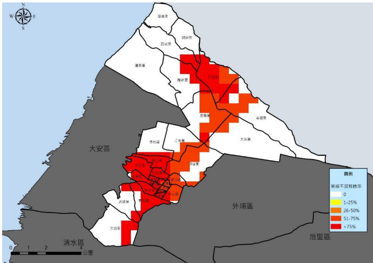
圖 1-3-11 大甲區危險物質管線不服務機率推估圖
