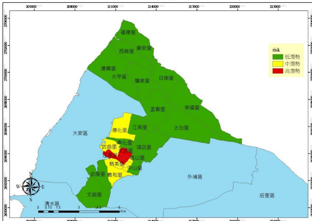
圖 1-3-25 大甲區 24 小時累積 650 毫米淹水潛勢圖
